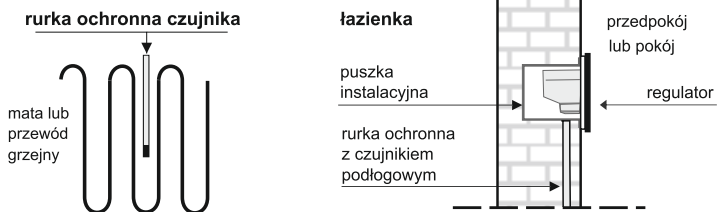
Do poprawnej instalacji czujnika podłogowego, zalecamy zakup specjalnej rurki ochronnej i luku prowadzącego.
