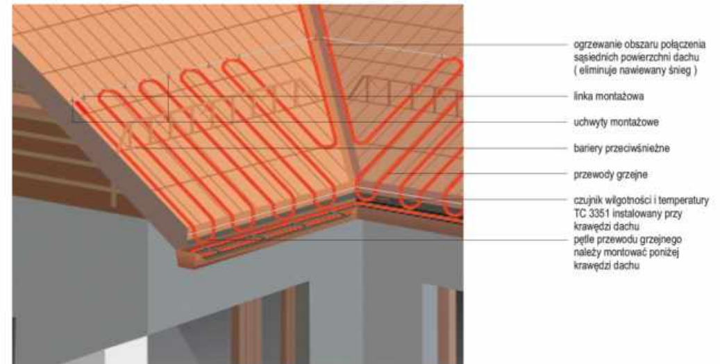
ogrzewanie strefy brzegowej dachu
