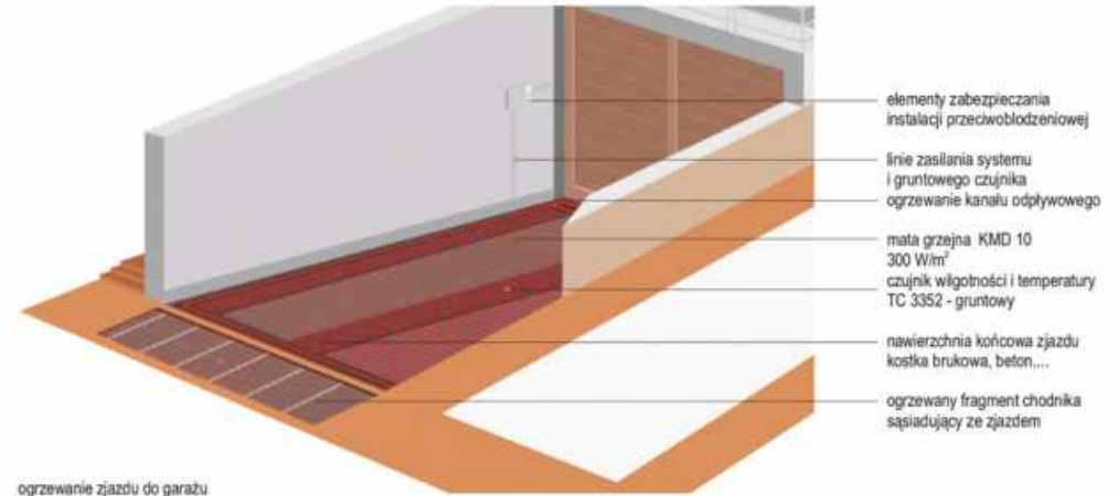
ogrzewanie zjazdu do garażu
