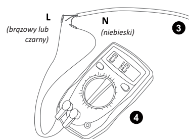
Pomiar rezystancji żyły grzejnej
