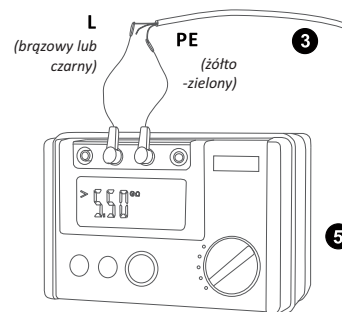
Pomiar rezystancji izolacji
